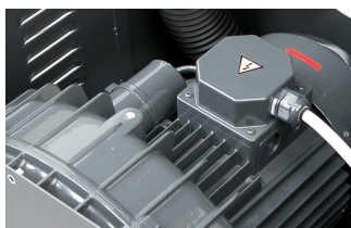
Moteur à turbine silencieux IP 55 et soupape de surpression incorporée
